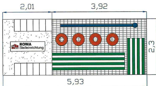
Abbildung 1: Grundplan der Mobilen Ställe ROWA 100 & 150, © ROWA Stalleinrichtung GmbH & Co. KG
