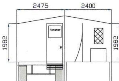
Abbildung 2: Außenansicht des Mobilsten Stalles ROWA 150 4.0, © ROWA Stalleinrichtung GmbH & Co. KG
