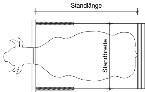
Abbildung 3: Vermessung der Standlänge und der Standbreite; © HBLFA Raumberg-Gumpenstein
