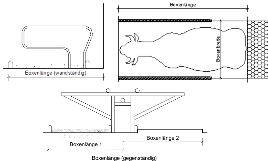
Abbildung 4: Vermessung von Liegeboxen; © HBLFA Raumberg-Gumpenstein
