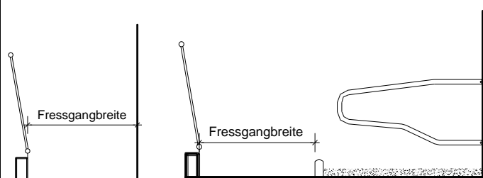
Abbildung 5: Vermessung der Fressgangbreite; © HBLFA Raumberg-Gumpenstein
