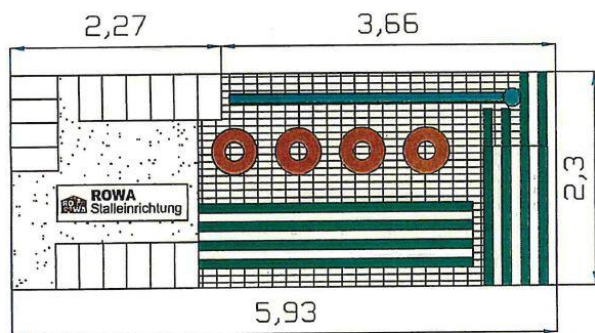
Grundplan des Mobilen Stalles ROWA 200
