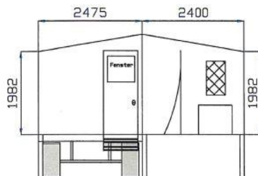
Außenansicht des Mobilen Stalles ROWA 200 4.0
